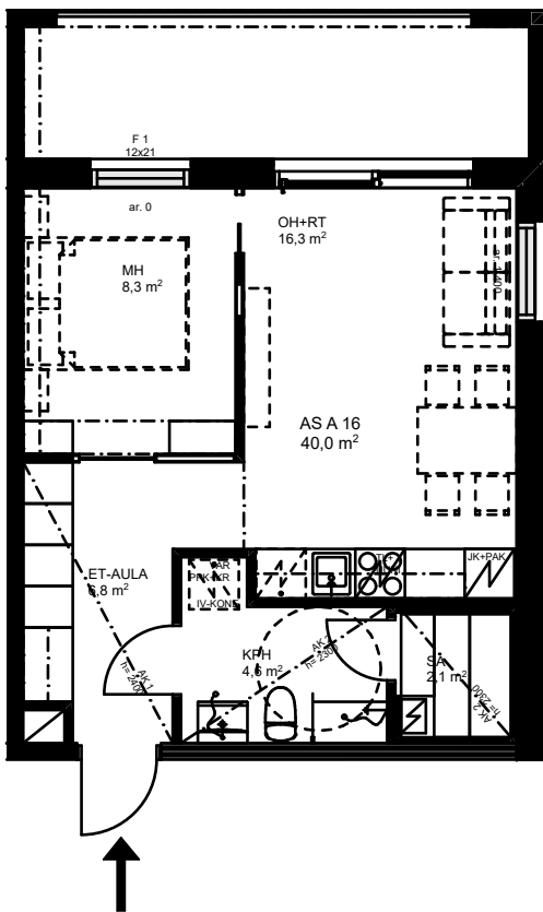
POHJAPIIRUSTUS 1:100
