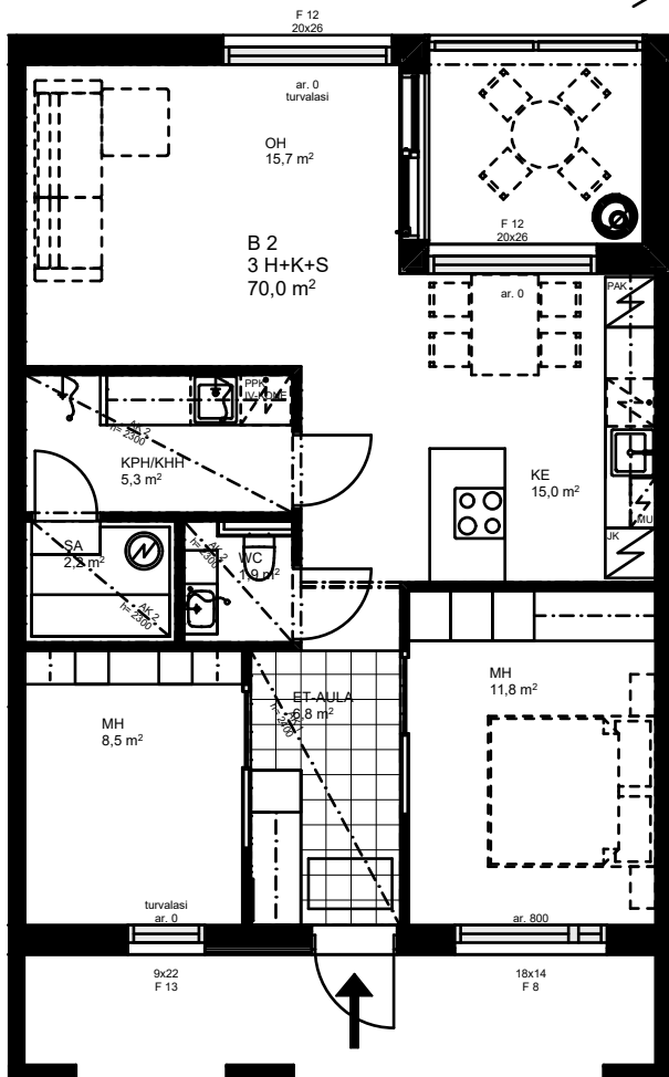
POHJAPIIRUSTUS 1:100
