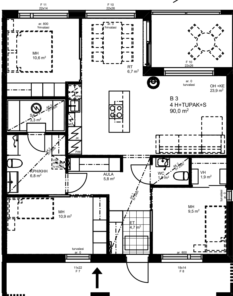
POHJAPIIRUSTUS 1:100
