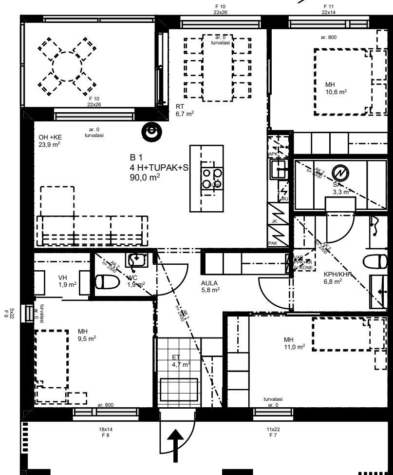
POHJAPIIRUSTUS 1:100
