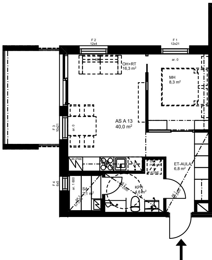
POHJAPIIRUSTUS 1:100
